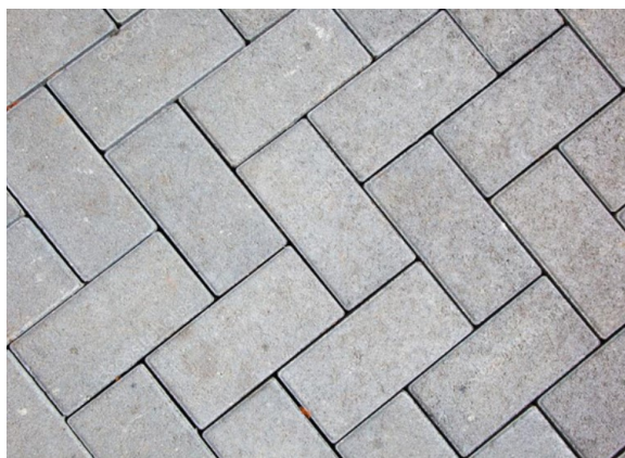
Figura 01. Forma de execução da instalação dos blocos intertravados em espinha de peixe das sarjetas com auxílio de guia de madeira
